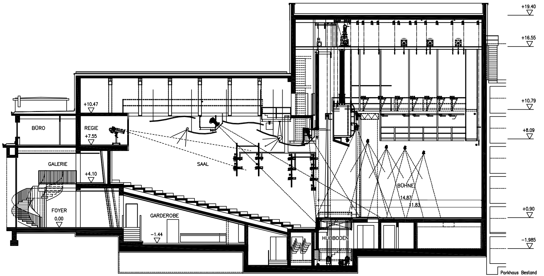
1 2 3 4 5 6 7 QUERSCHNITT M. 1:200
