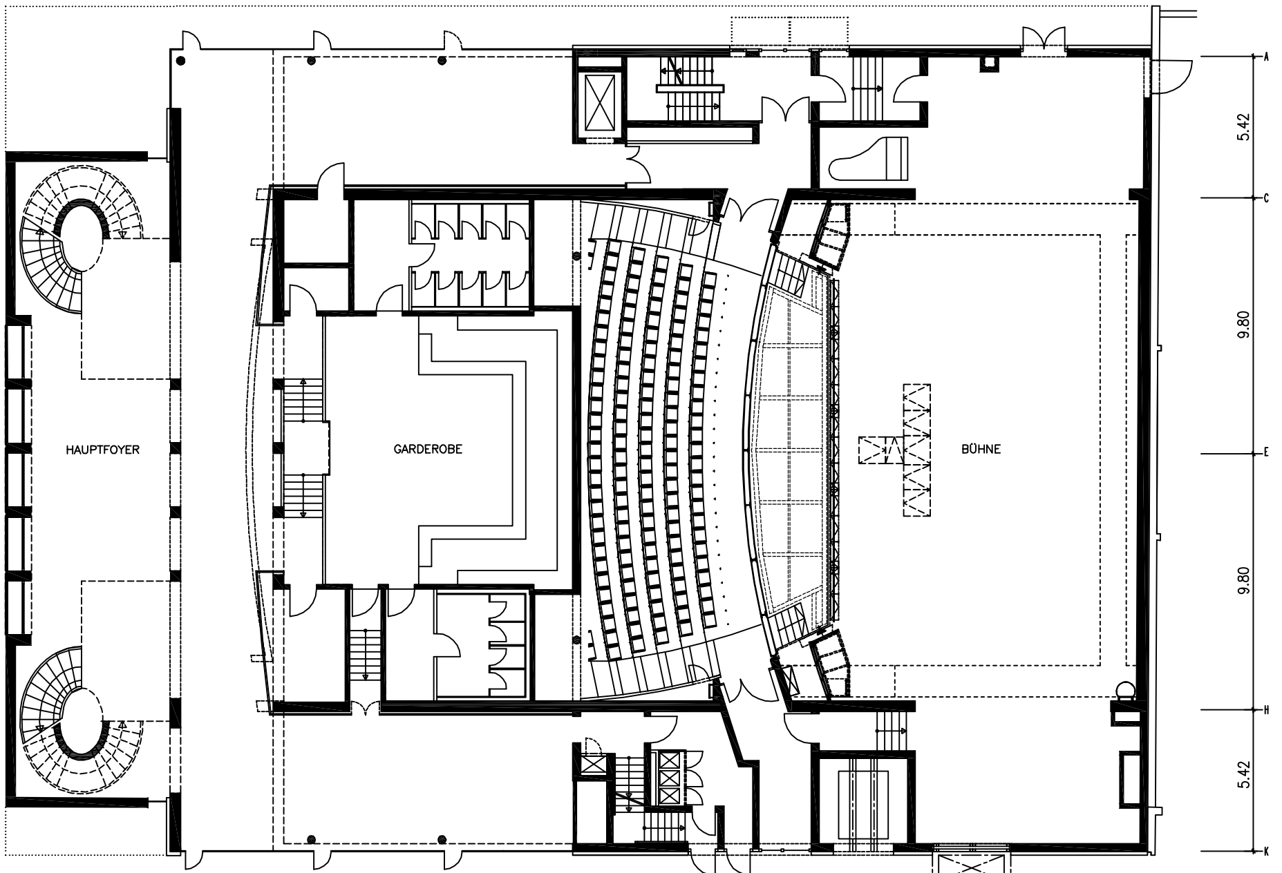
1 2 3 4 5 6 7 ERDGESCHOSS M. 1:200
